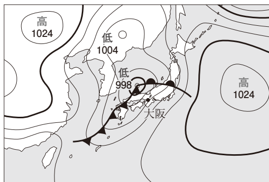
図2 4月14日21時の天気図
