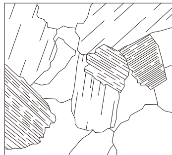
図2 火成岩のスケッチ
