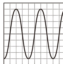
図2 音の波形
