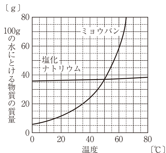
図４ 溶解度曲線
