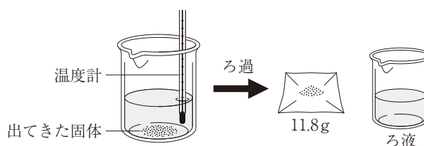
図3 ビーカー内のようすと、ろ過した後にとり出した固体とろ液のようす
